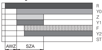
Anlauf ohne Flammenbildung Startup without flame generation Démarrage sans formation de flamme Avviamento senza formazione fiamme
