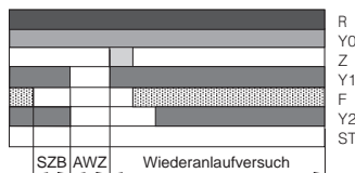
Flammenausfall während des Betriebes mit Wiederanlauf Flame failure during operation with restart Perte de flamme en cours de fonctionnement avec redémarrage Mancanza di fiamma durante l'esercizio con riavvio
