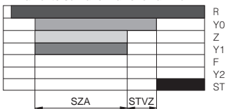
Anlauf ohne Flammenbildung Startup without flame generation Démarrage sans formation de flamme Avviamento senza formazione fiamme
