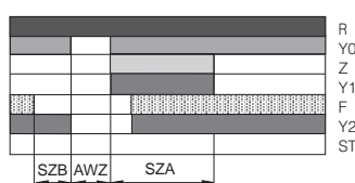
Flammenausfall während des Betriebes mit Wiederanlauf Flame failure during operation with restart Extincion de la flamme en cours de fonctionnement avec redémarrage Mancanza di fiamma durante l'esercizio con riavvio
