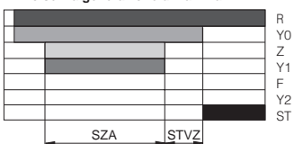
Anlauf ohne Flammenbildung Startup without flame formation Démarrage sans formation de flamme Avvio senza generazione di fiamma
